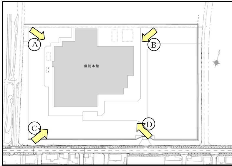
Ⓑ 3・4階柱・梁完了
